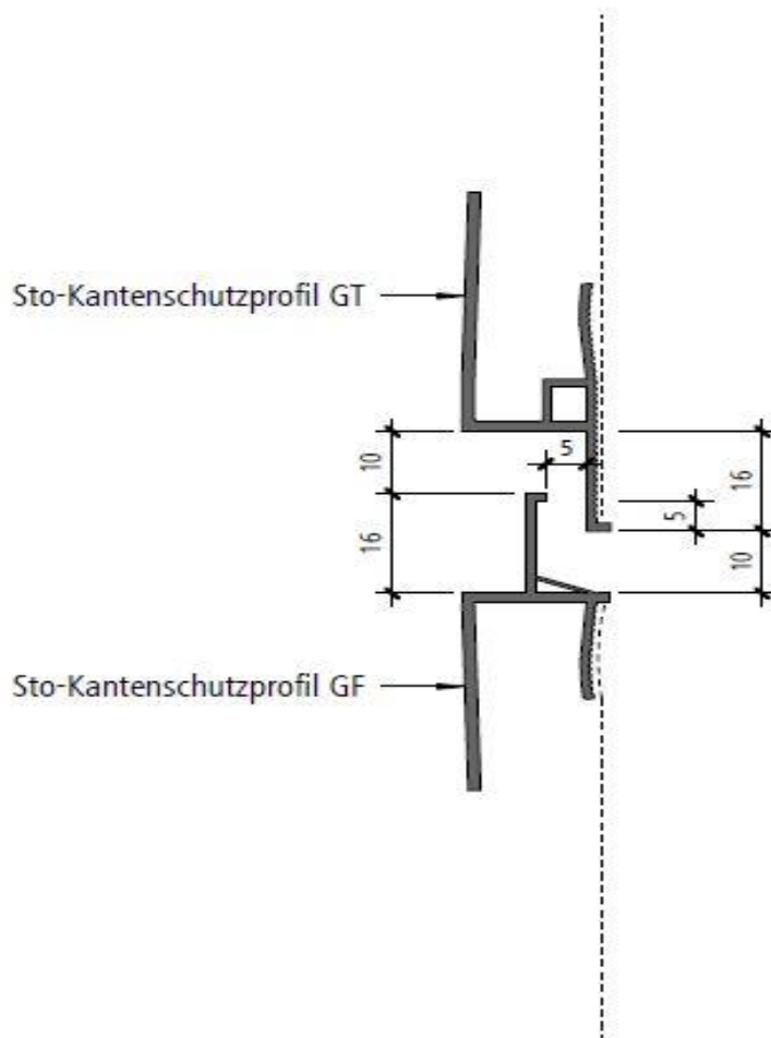
varijanta StoProfile Edge GT/GF
